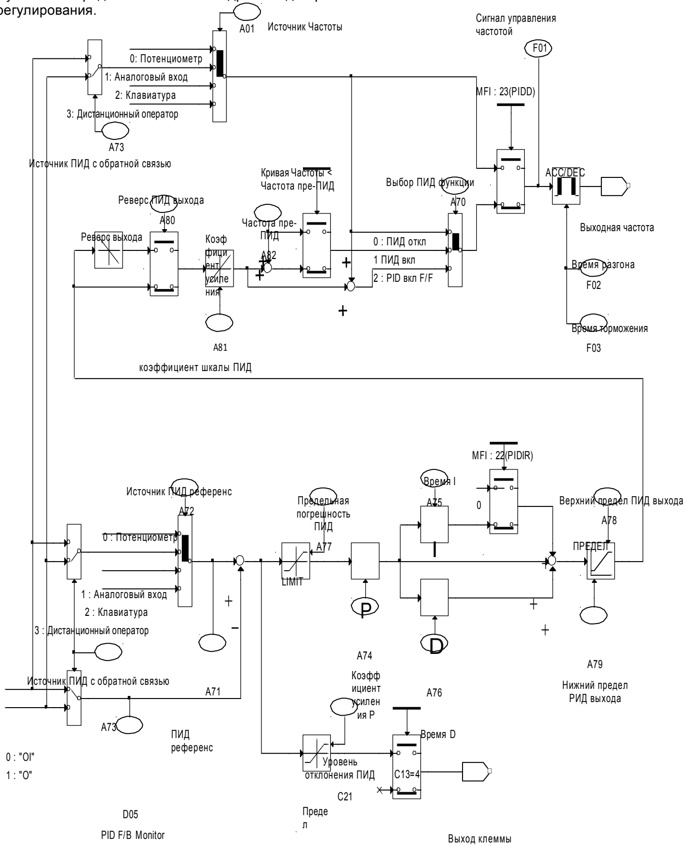
Рис 4-1 Диаграмма ПИД
