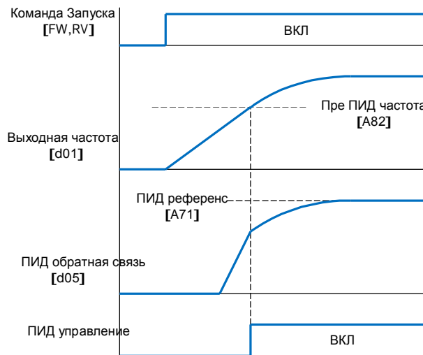
Рис 4-2 Пре-ПИД
